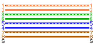
ワイヤーマップ: T568B
